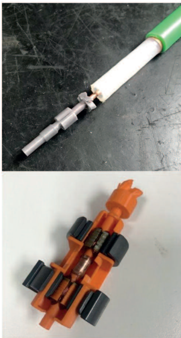
Interacció de la solució amb el cable coaxial i prototip final.
