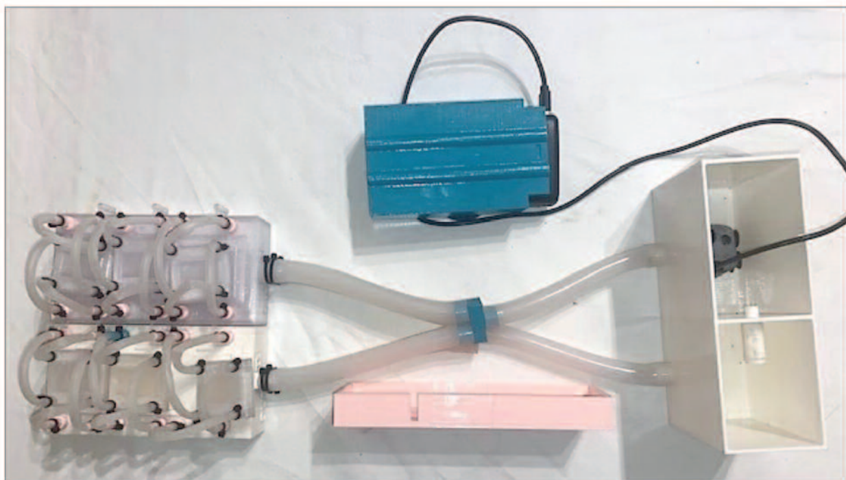
Muntatge del circuit en mode bioreactor utilitzant 2 mòduls de canals.
